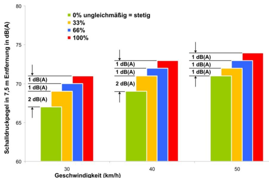
Abbildung 4: Lärminderungspotenzial durch Geschwindigkeitsreduzierung und Verstetigung des Verkehrsflusses
